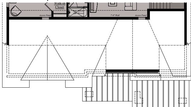
Elevation C - Optional Loft Level
